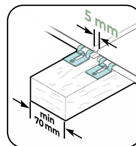
Lambourde de largeur > 70 mm + clips simples
